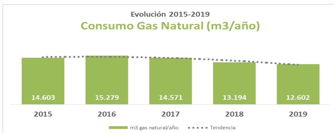
Ilustración 10 Evolución del consumo de gas natural
